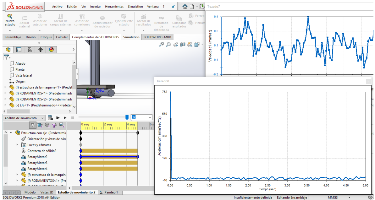
Ilustración 47. Análisis dinámico de rodamientos, disparo de motor hidráulico.
