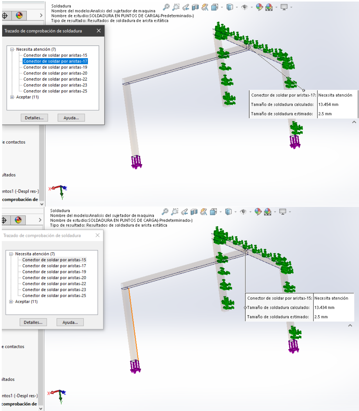
Ilustración 37. Análisis de soldadura con cargas segundo punto crítico en portería de la estructura.
