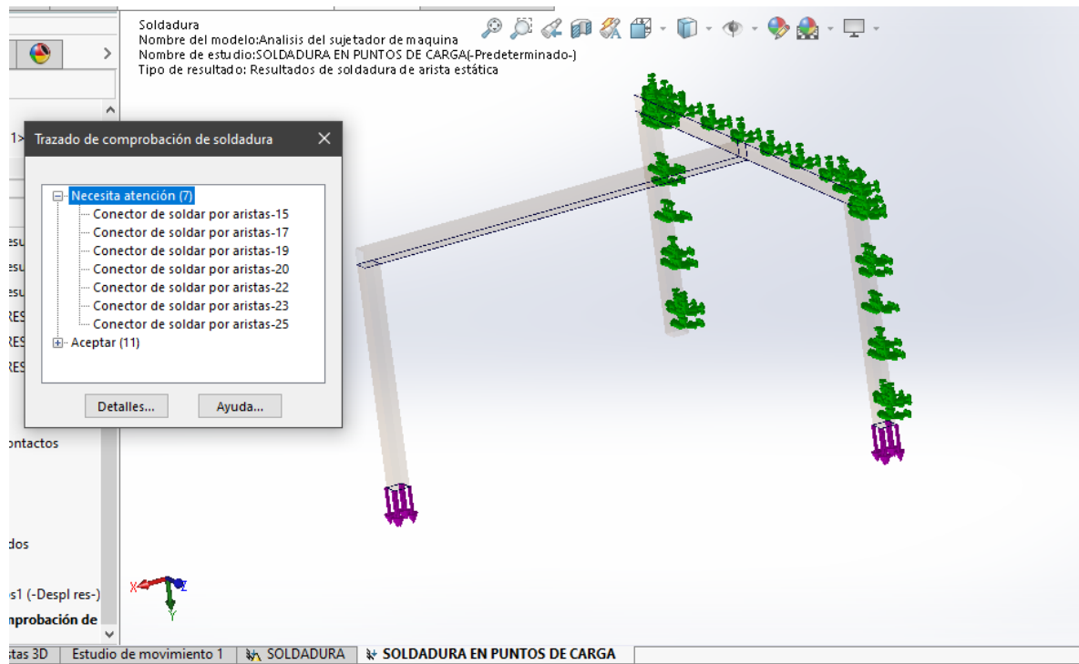
Ilustración 36. Análisis de soldadura con cargas primer punto crítico en portería de la estructura.
